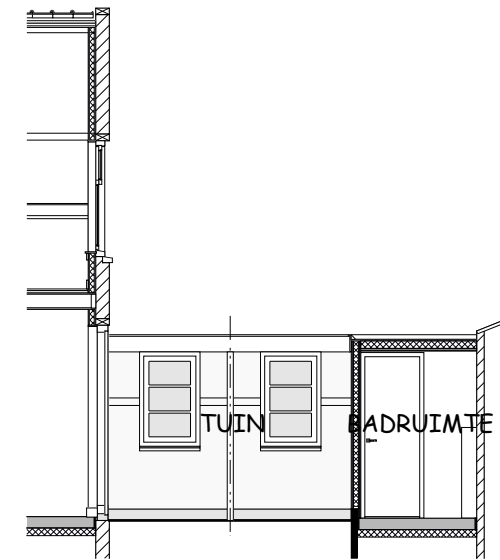
LINKER ZIJGEVEL
