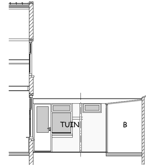
LINKER ZIJGEVEL
