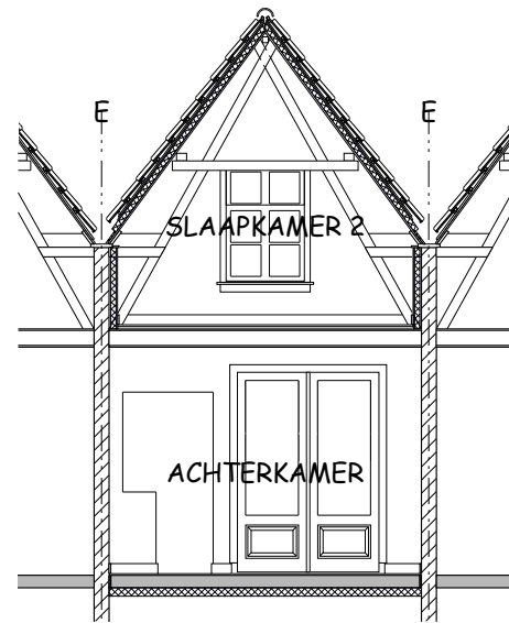
DWARSDOORSNEDE
