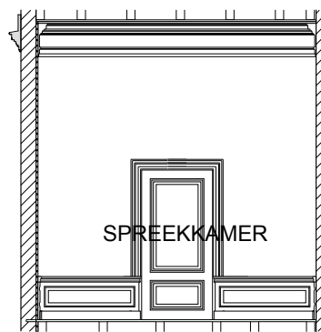
WAND KANTOORRUIJTE
