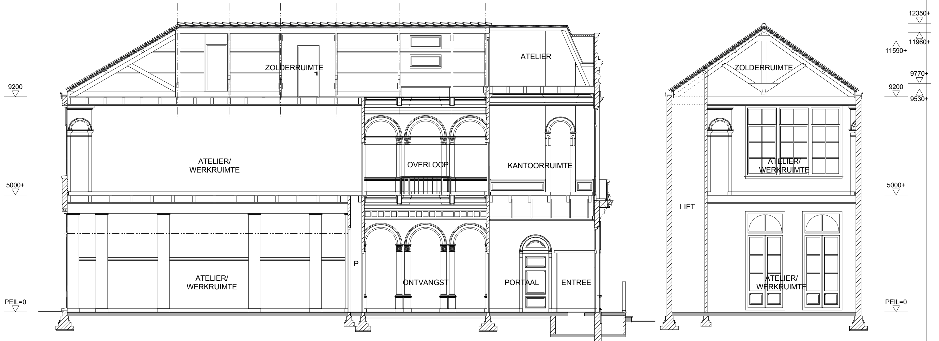
LANGSDOORSNEDE
